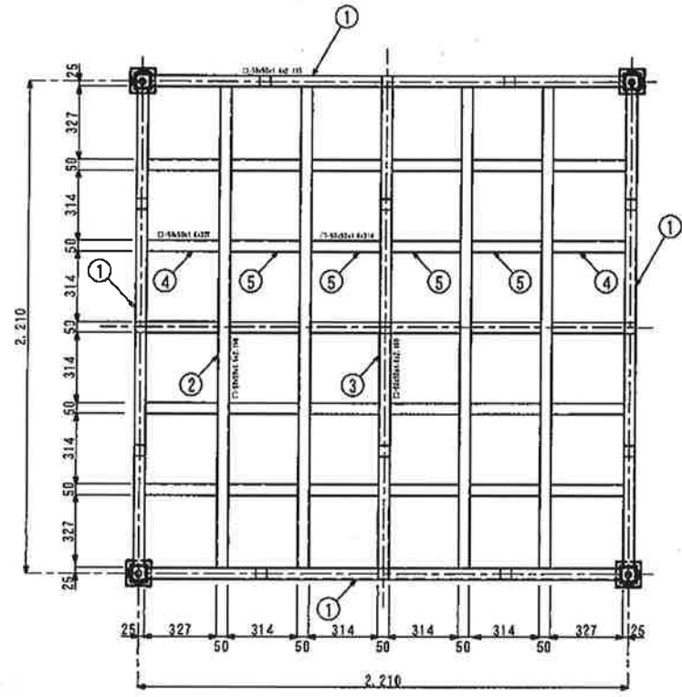
床面別見る S=1/15
