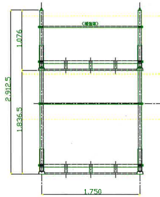
側面図 S=1/5
