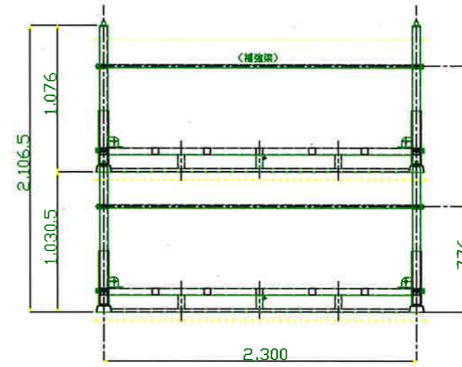
正面図 S=1/5
