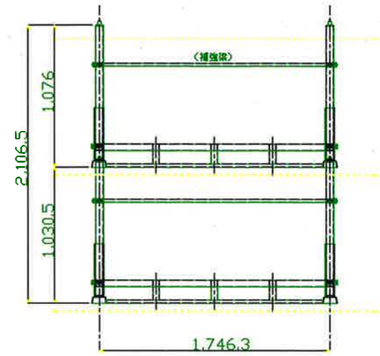
側面図 S=1/5
