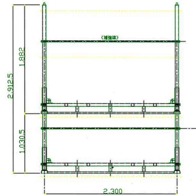
正面図 S=1/5
