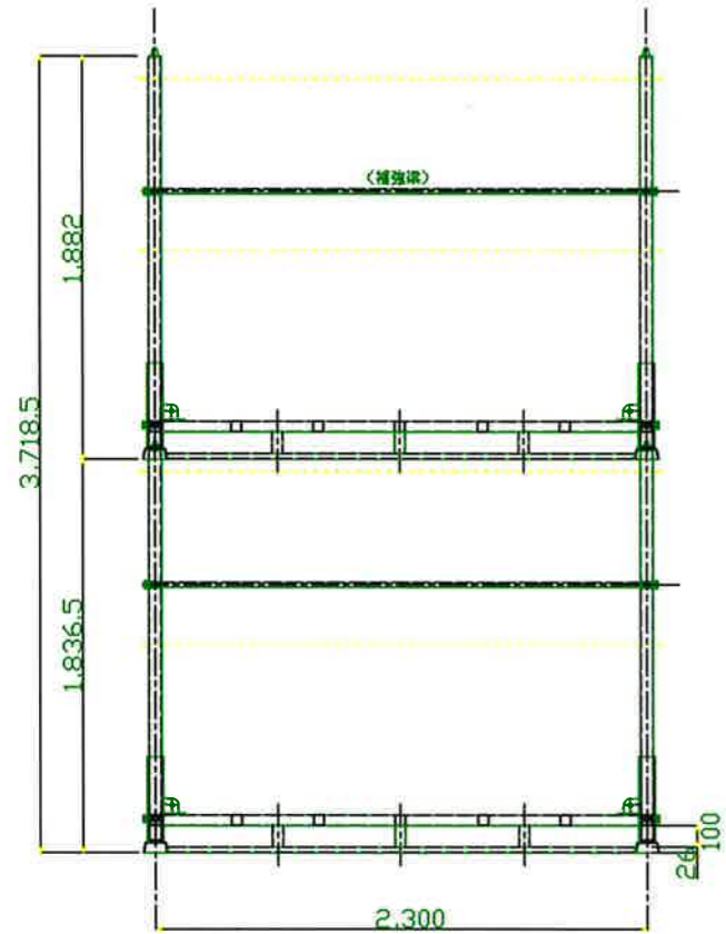
正面図 S=1/5
