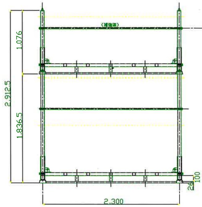
正面図 S=1/5
