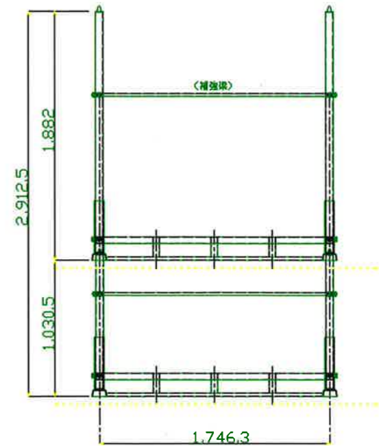
側面図 S=1/5
