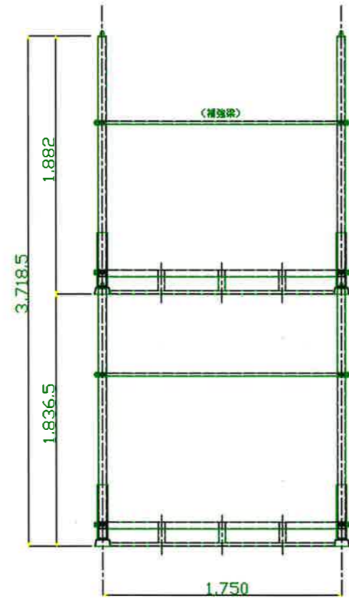
側面図 S=1/5
